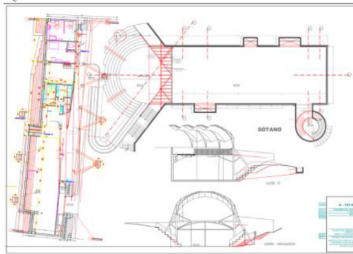
Plano de planta: estructura metálica, geomembrana y sistema de recolección de agua de lluvia
