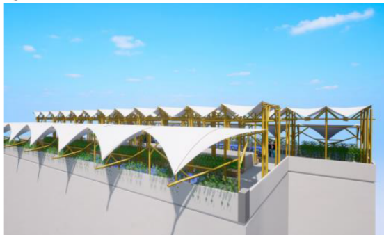
Vista exterior: estructura de bambú, membrana geotextil.
