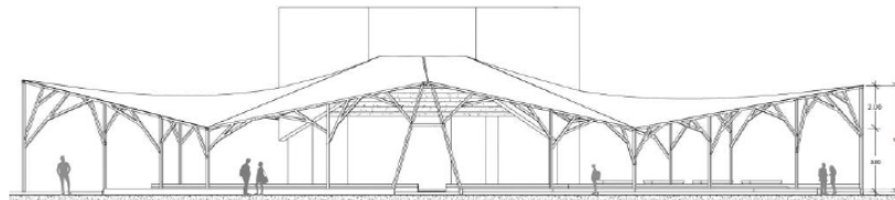
Plano de corte: fachada del proyecto con tensionada y estructura de acero
