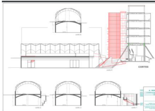
Cortes y elevaciones: estructura metálica, geomembrana y sistema de recolección de aguas de lluvia
